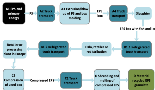
Figur 1: Flytskjema som viser systemgrensene
